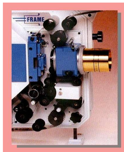
Passaggio film - Threading assembly - Mecanisme d'entrainement
